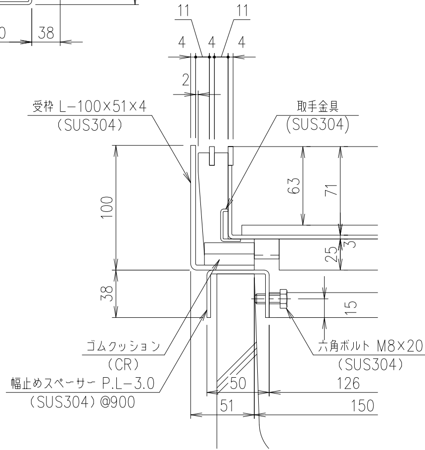
部分詳細図 S=1/3
