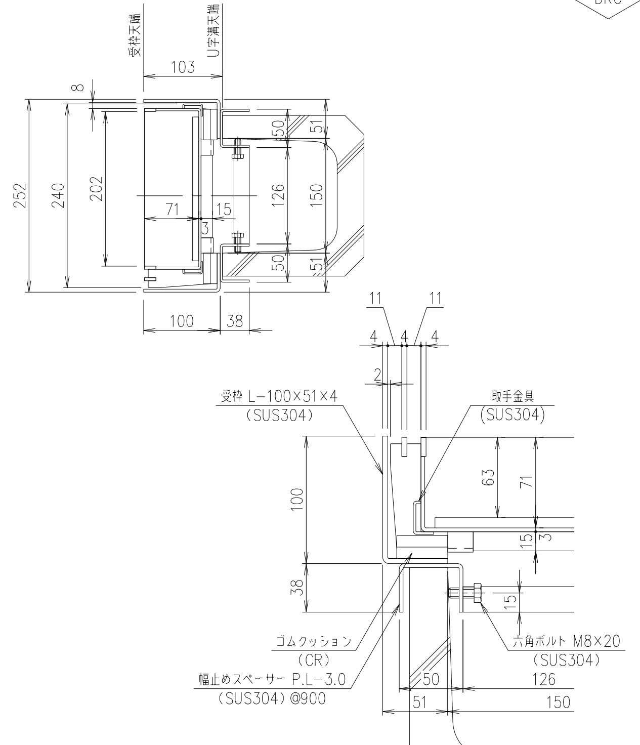
部分詳細図 S=1/3
