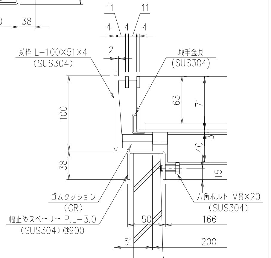
部分詳細図 S=1/3
