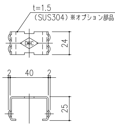
ボルト穴カバー：(特)CAP-19 詳細図 S=1/2 ※オプション部品
