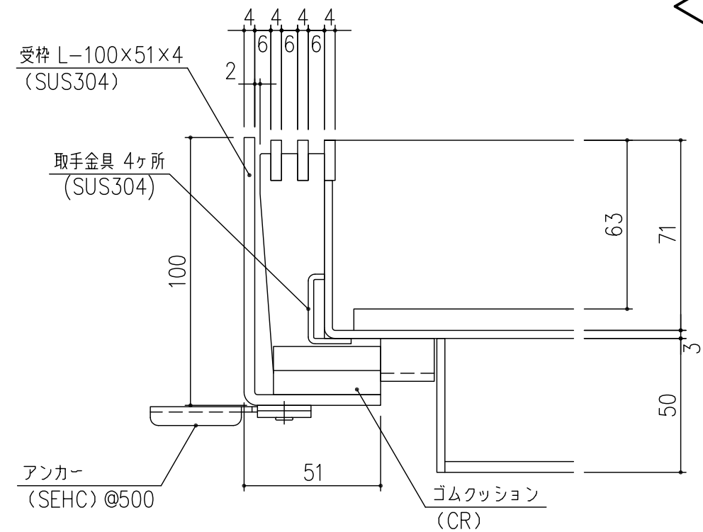
A部 詳細図 S=1/2
