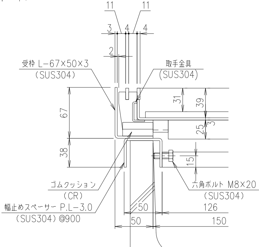
部分詳細図 S=1/3
