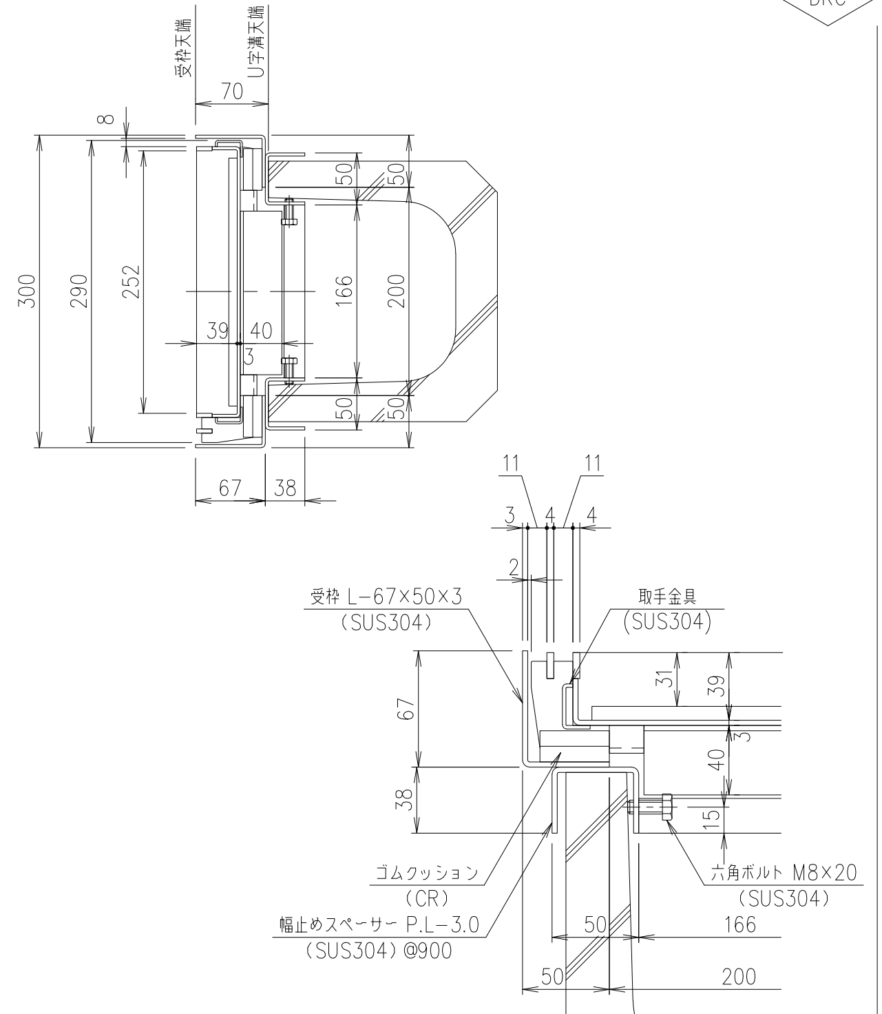
部分詳細図 S=1/3
