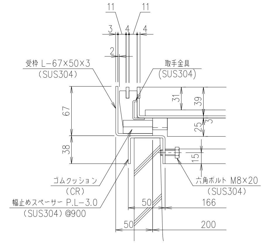
部分詳細図 S=1/3
