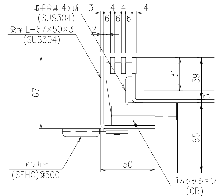
A部詳細図 S=1/2
