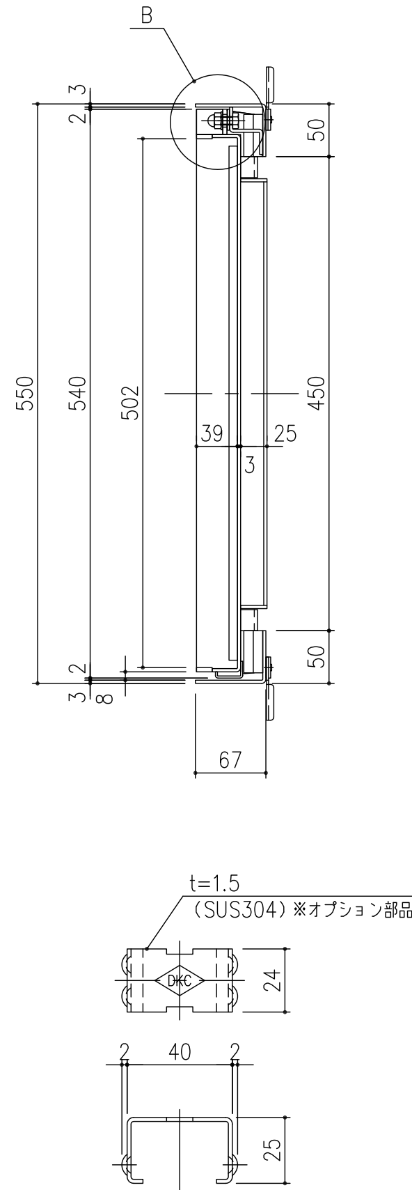
ボルト穴カバー：(特)CAP-19 詳細図 S=1/2 ※オプション部品
