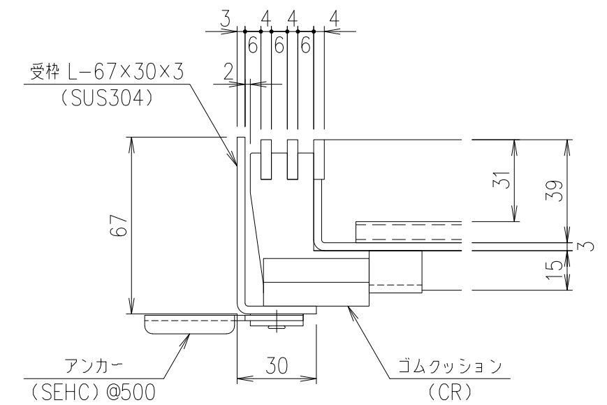
A部 詳細図 S=1/2
