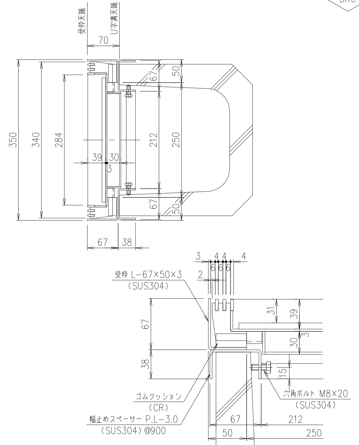
部分詳細図 S=1/3
