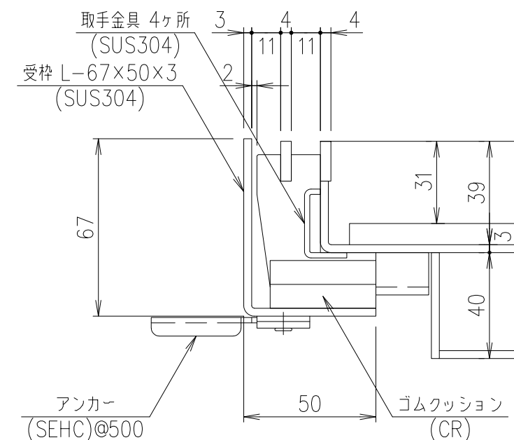
A部詳細図 S=1/2
