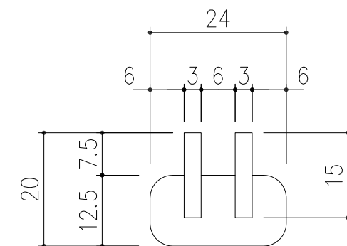
蓋詳細圖 S=1/1
