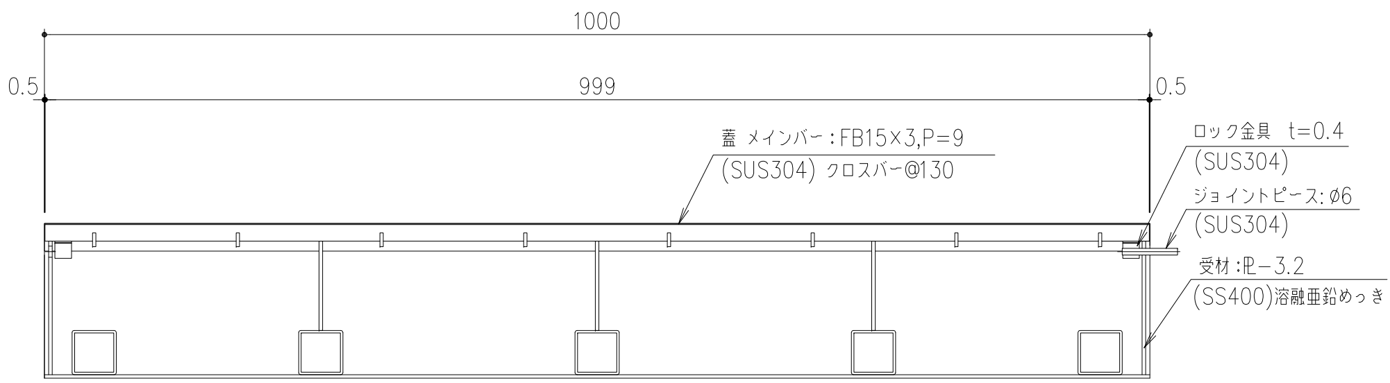
断面：A-A
