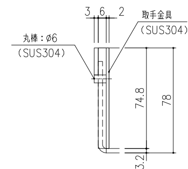
取手金具 詳細図 S=1/2
