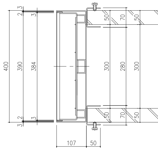
断面: A-A
