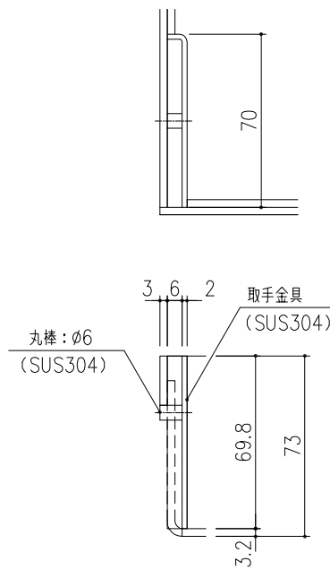
取手金具 詳細図 S=1/2
