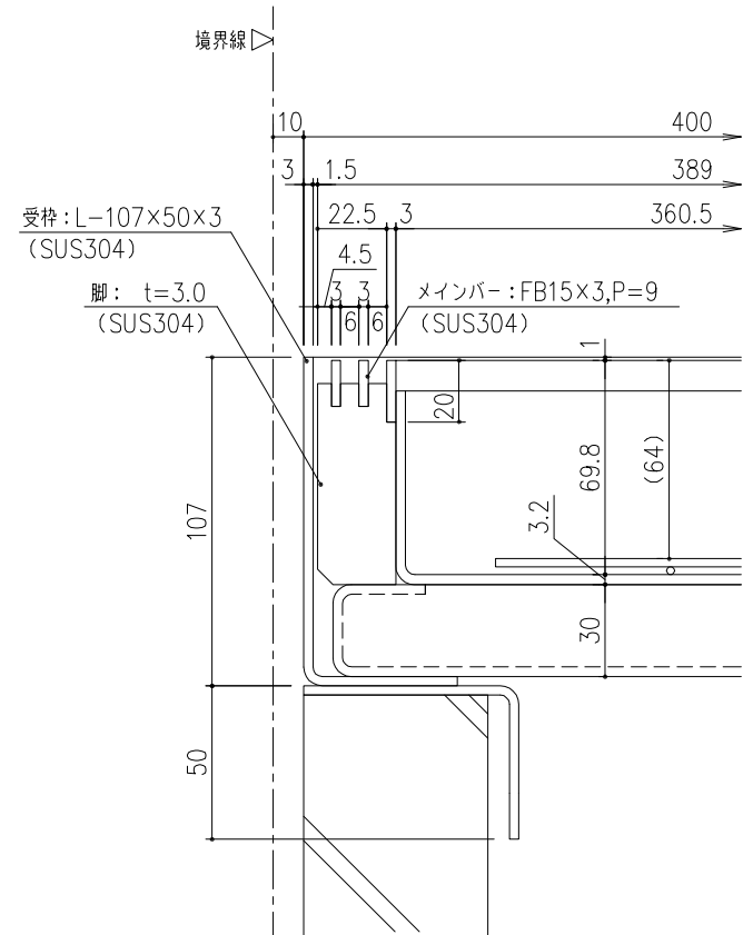
スリット部断面詳細図 S=1/2
