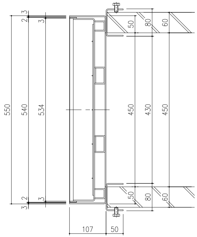
断面: A-A
