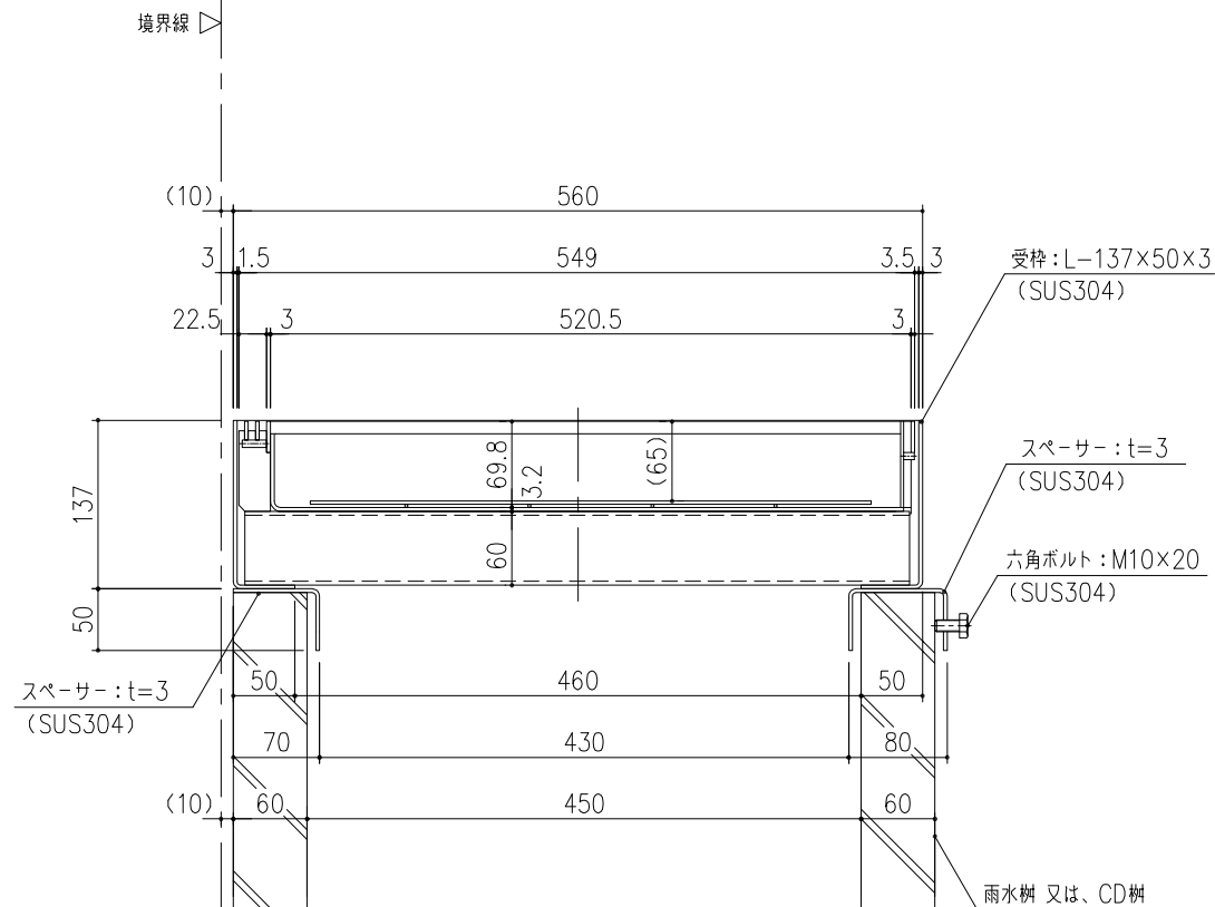
断面：B-B
