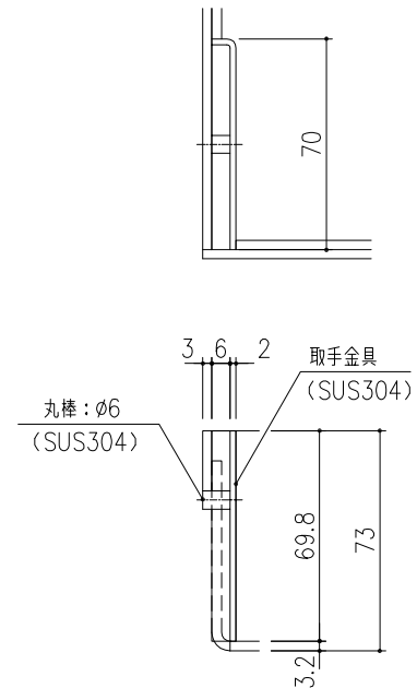
取手金具 詳細図 S=1/2
