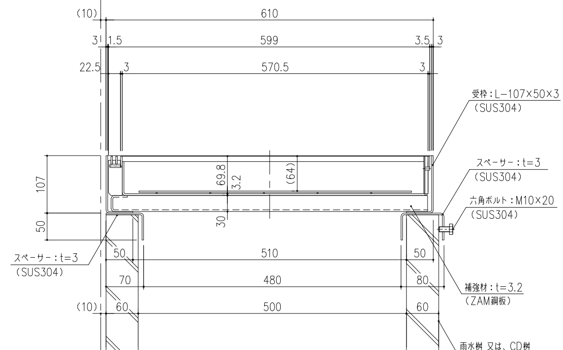
断面: B-B
