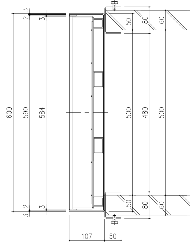
断面: A-A
