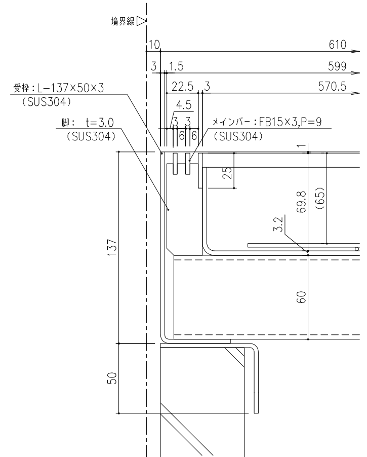
スリット部断面詳細図 S=1/2
