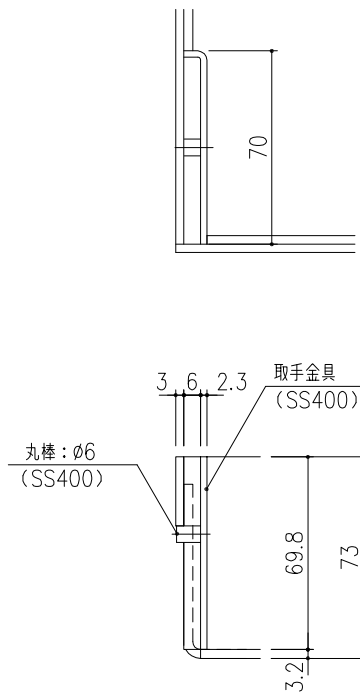
取手金具 詳細図 S=1/2
