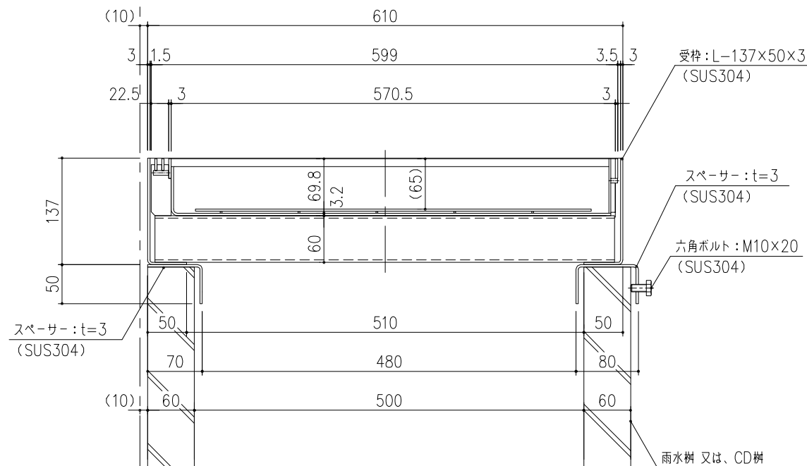
断面：B-B
