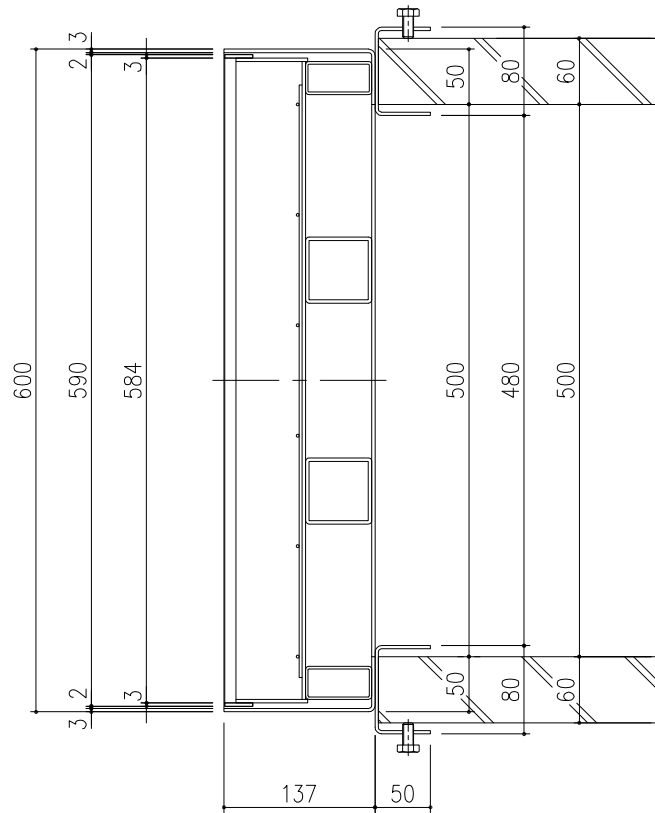
断面：A-A
