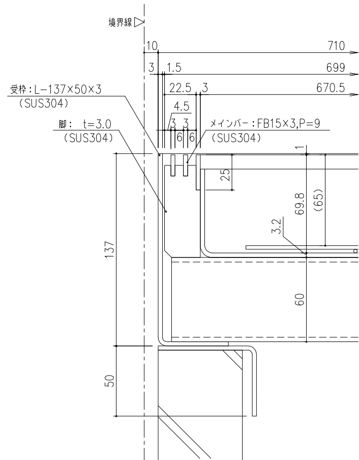
スリット部断面詳細図 S=1/2
