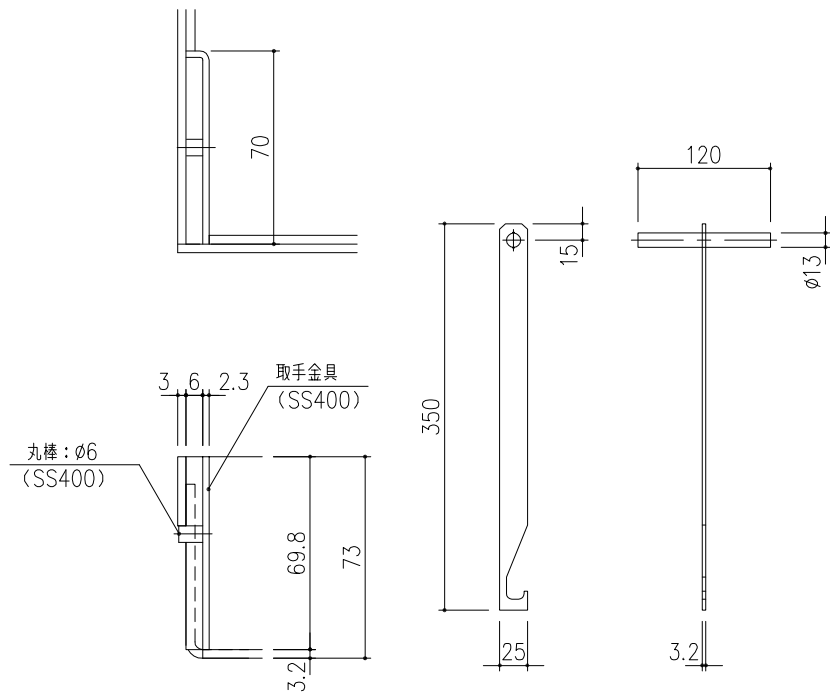
取手金具 詳細図 S=1/2
