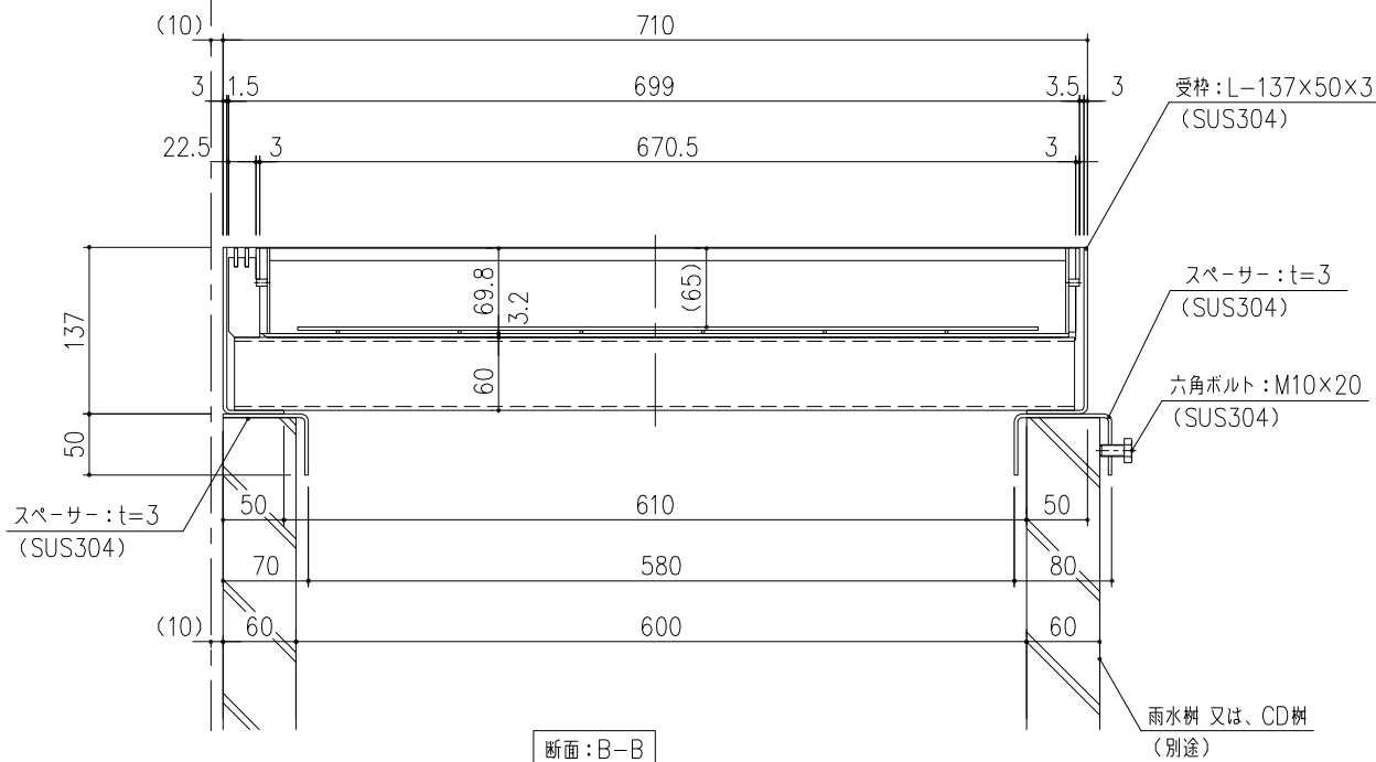
断面：B-B
