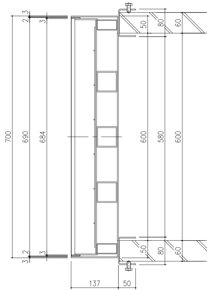
断面：A-A
