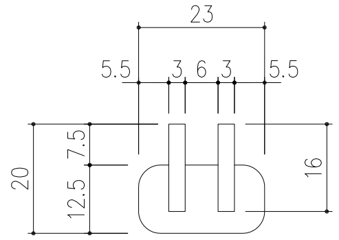
蓋詳細図 S=1/1
