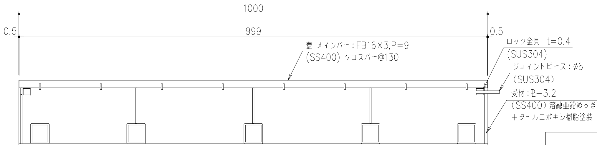
断面 : A-A
