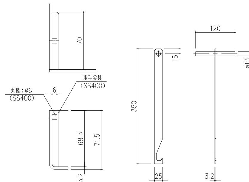
取手金具 詳細図 S=1/2
