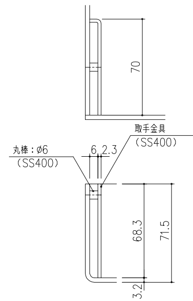
取手金具 詳細図 S=1/2
