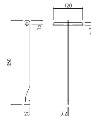
オプション：開閉フック（MF-62） （S45C）電気垂鉛めっき
