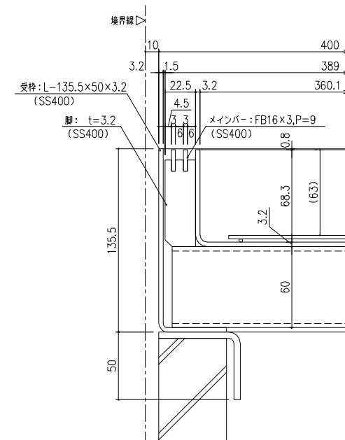
スリット部断面詳細図 S=1/2
