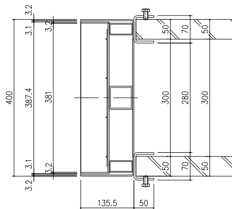
断面：A—A
