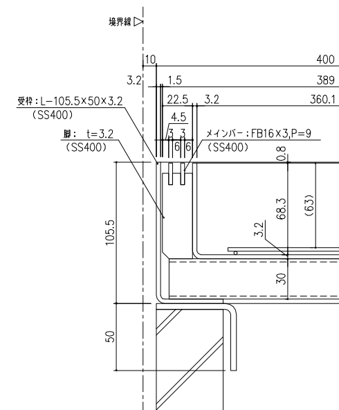
スリット部断面詳細図 S=1/1
