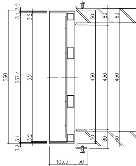
断面：A-A
