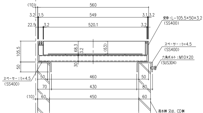
断面：B-B
