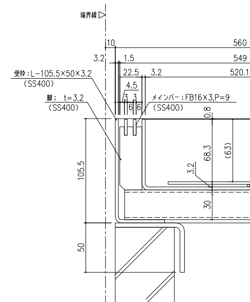
スリット断面詳細図 S=1/2
