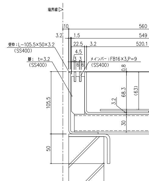
スリット部断面詳細図 S=1/2
