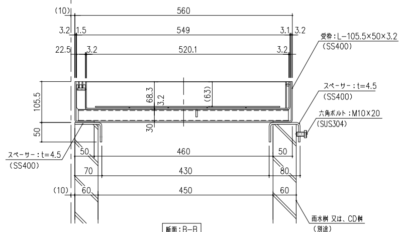
断面：B—B
