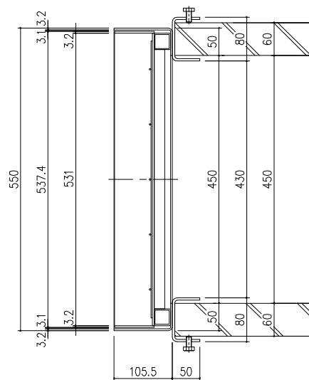
断面：A—A
