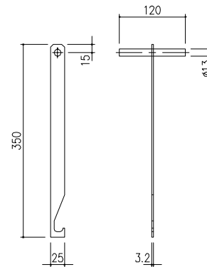
オプション: 開閉フック (MF-62) (S45C) 電気溶接めっき
