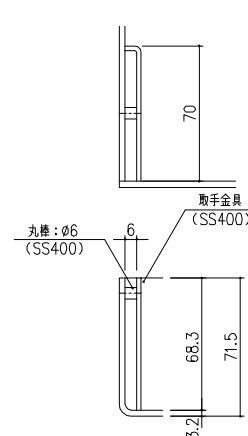
取手金具 詳細図 S=1/2
