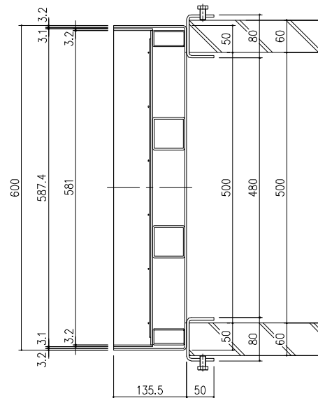
断面：A—A
