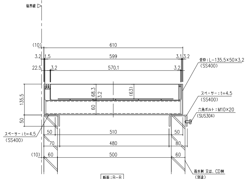
断面：B-B
