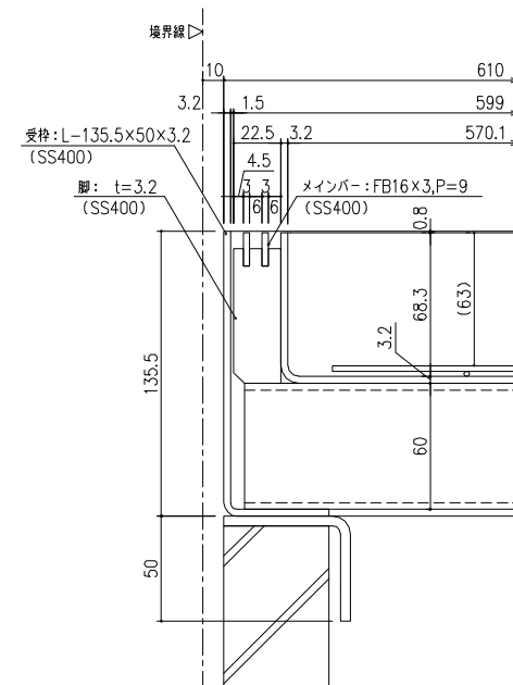
スリット部断面詳細図 S=1/2
