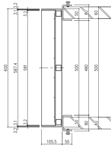
断面：A-A
