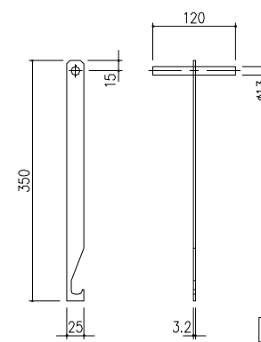
オプション：開閉フック (MF-62) (S45C) 電気配線用
