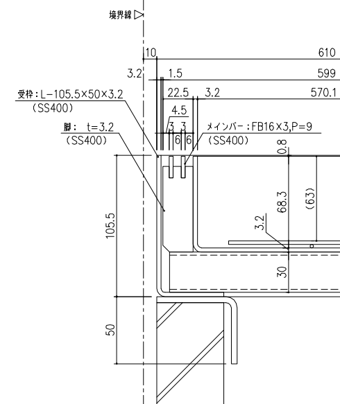
スリット断面詳細図 S=1/2
