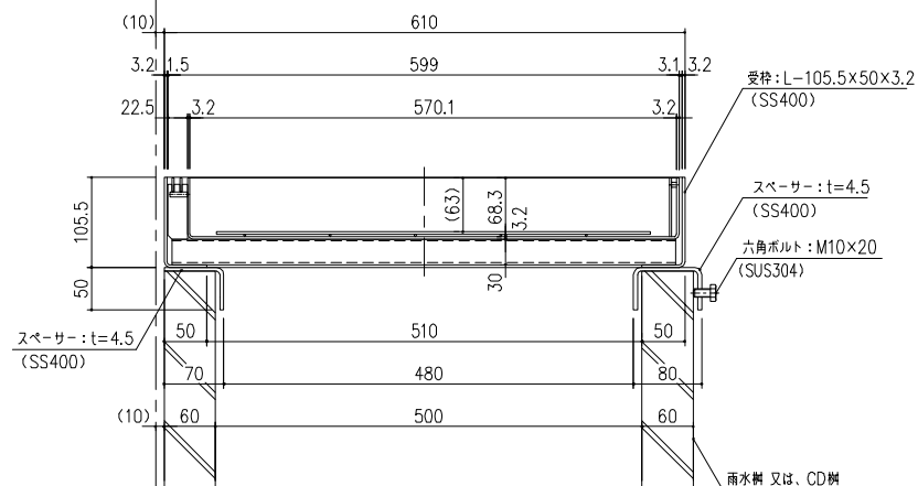
断面：B-B
