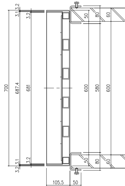
断面: A-A
