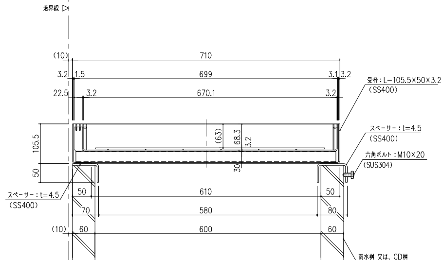
断面: B-B
