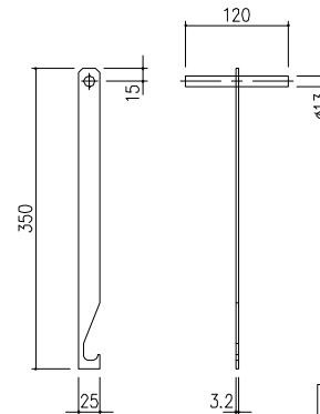
オプション: 開閉フック (MF-62) (S45C) 電気面鉛めっき
