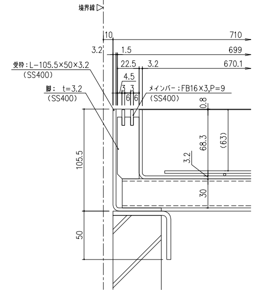
スリット断面詳細図 S=1/2
