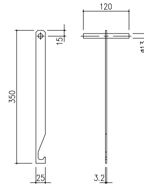
オプション：開閉フック (MF-62) (S45C) 電気絶縁めっき
