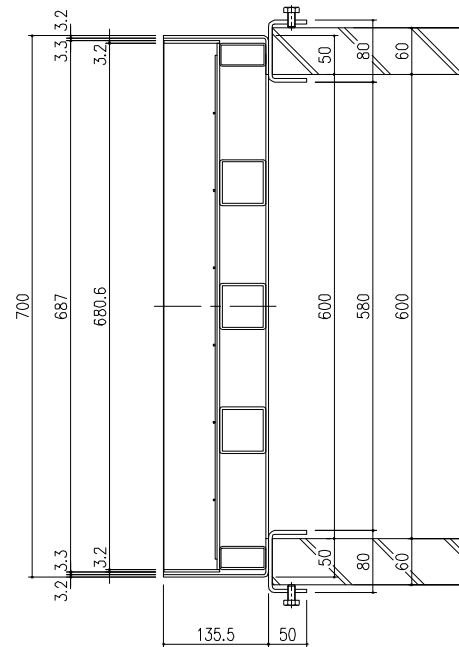
断面：A-A
