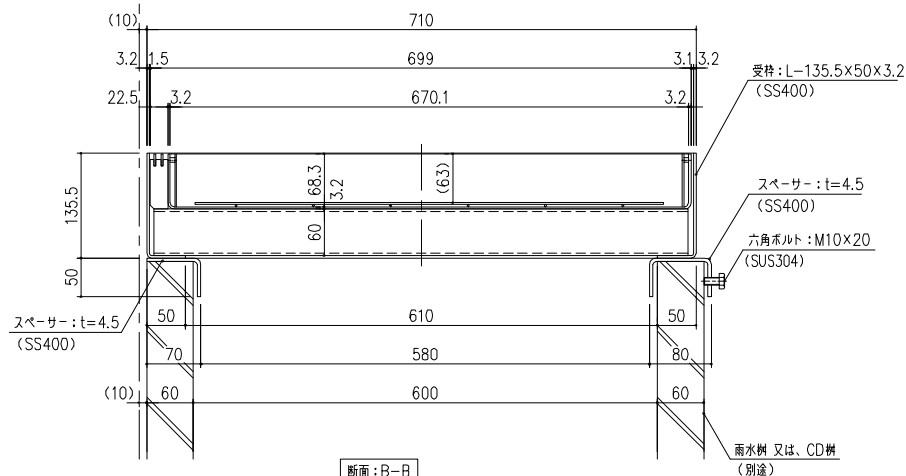
断面：B-B
