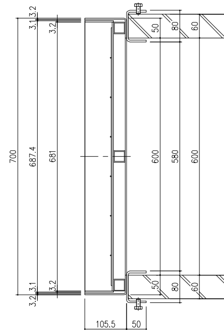
断面：A—A
