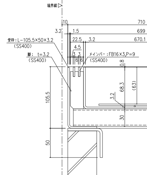
スリット部断面詳細図 S=1/2
