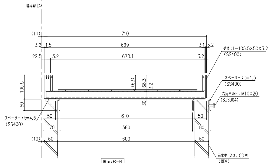
断面: B-B
