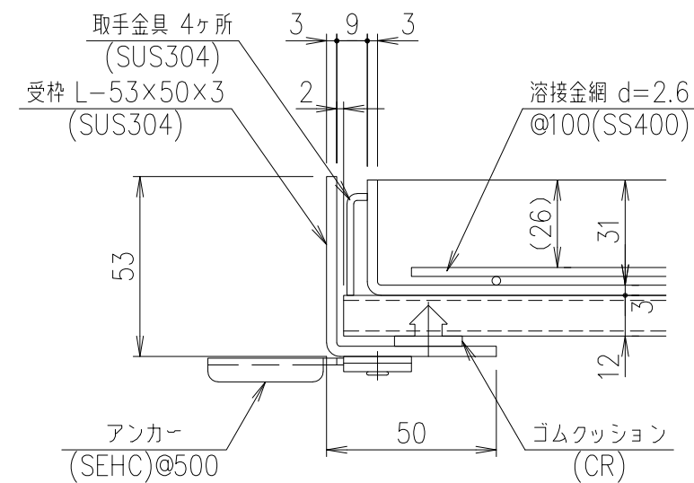
A部詳細図 S=1/2
