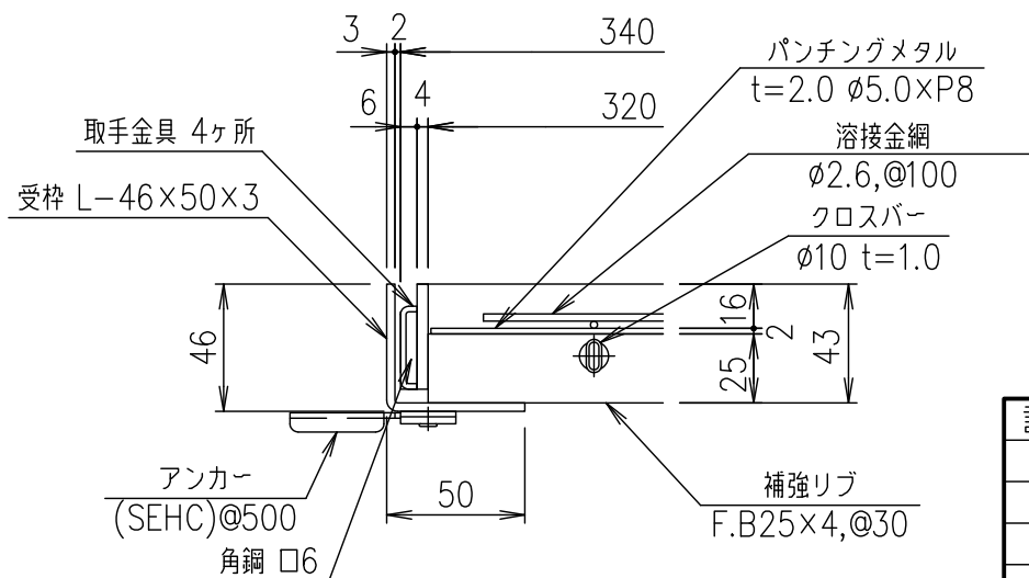
部分詳細図 S=1/3
