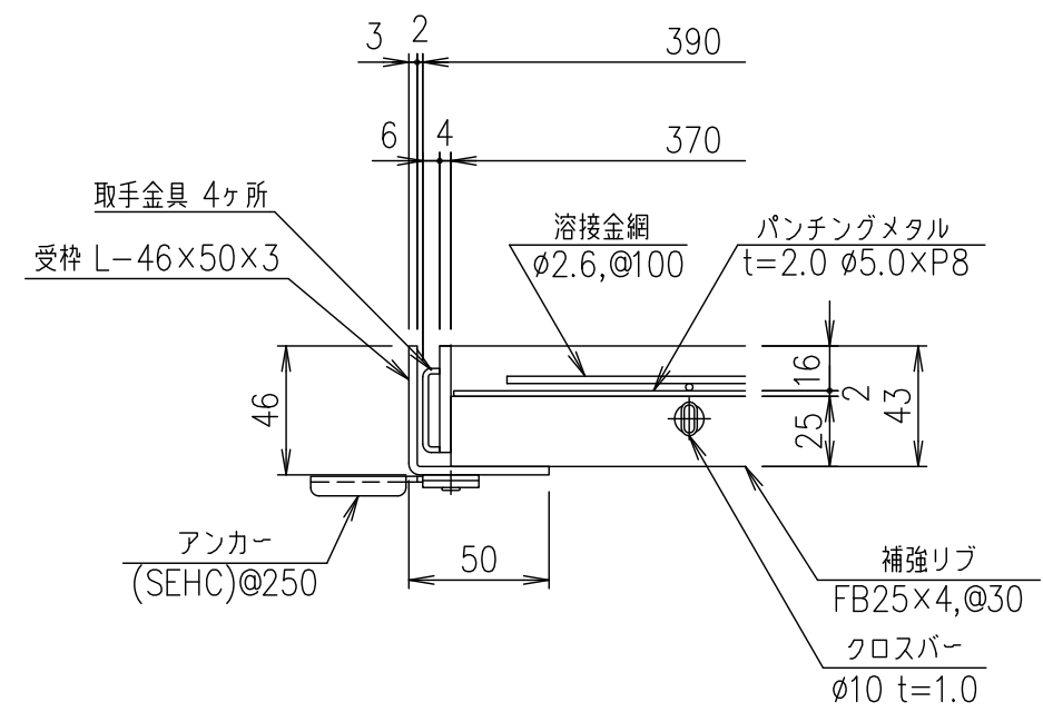
部分詳細図 S=1/3
