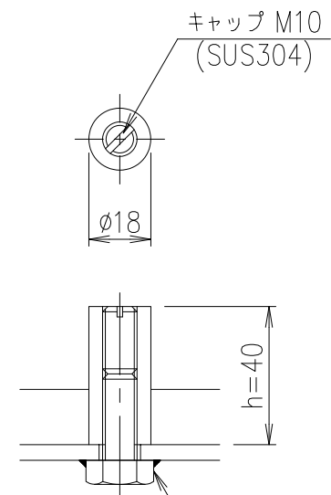
部分詳細図 S=1/3
