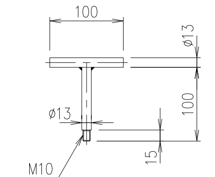
開閉ハンドル S=1/5 SS400,電気垂鉛めっき
