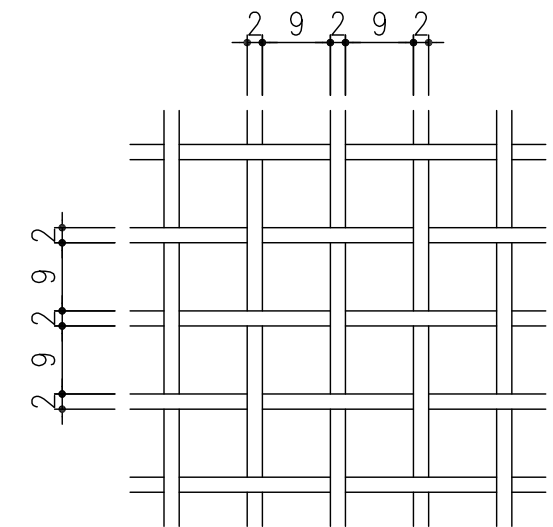
クリンプ金網 線径φ2.0、開き目9 S=1/1
