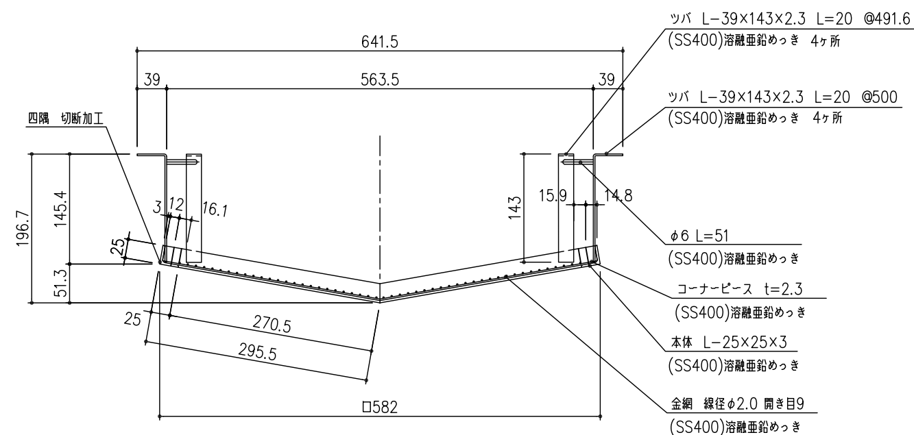
ZLSC-ET 600 平面・断面詳細図 S=1/5 リーブスクリーン
