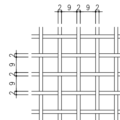
クリンプ金網 線径φ2.0、開き目9 S=1/1
