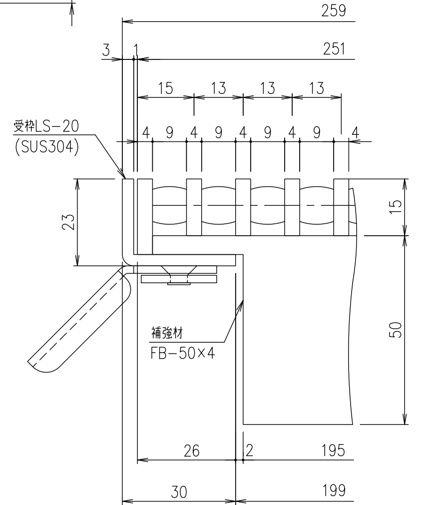
受枠断面・メインバーピッチ詳細図 S=1/1
