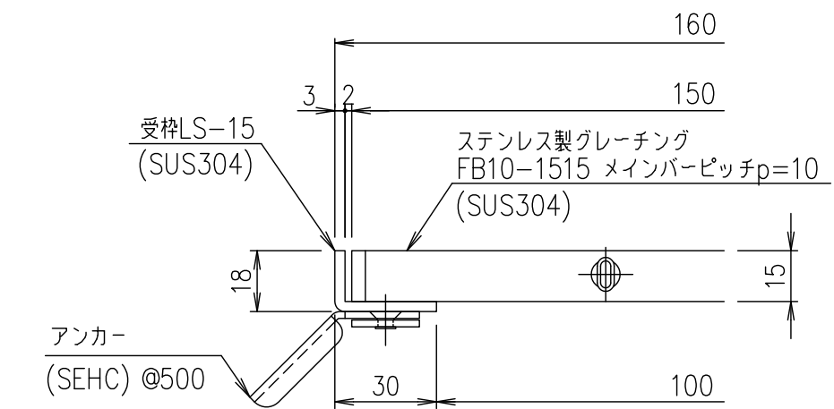
受枠断面詳細図 S=1/2
