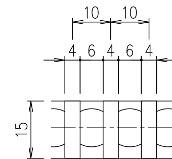
メンバーピッチ詳細図 S=1/1
