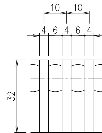
メインバーピッチ詳細図 S=1/1
