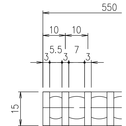
メインバーピッチ詳細図 S=1/1
