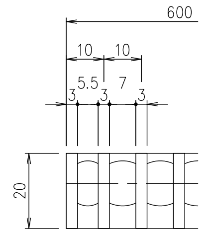
メインバーピッチ詳細図 S=1/1
