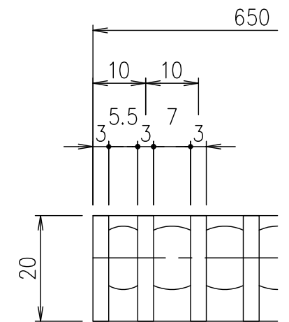
メンバーピッチ詳細図 S=1/1
