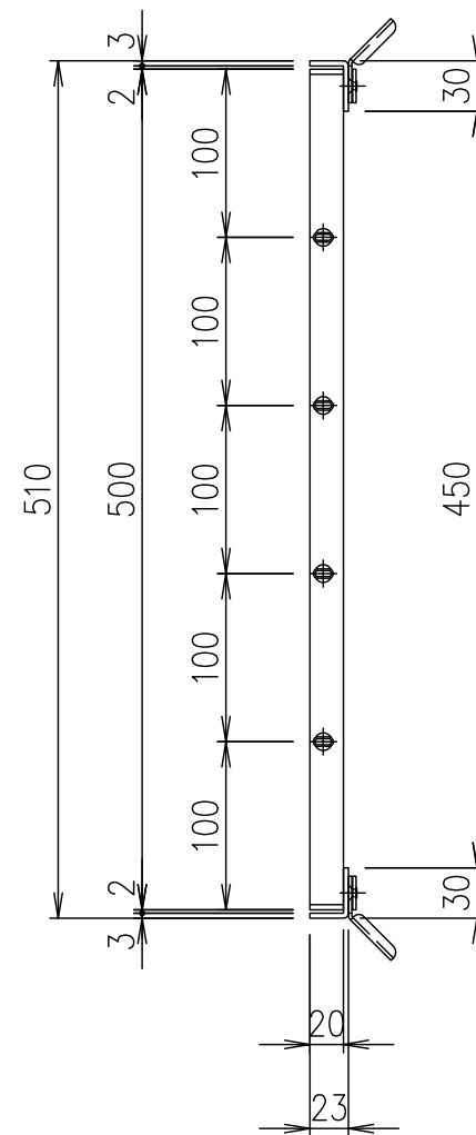
受枠LSM-20 (SUS304) ステンレス製グレーチングますぶた FBEM13-2050 メインバーピッチ p=13 (SUS304) アンカー (SEHC) □510 □500 23 30 20 □450
